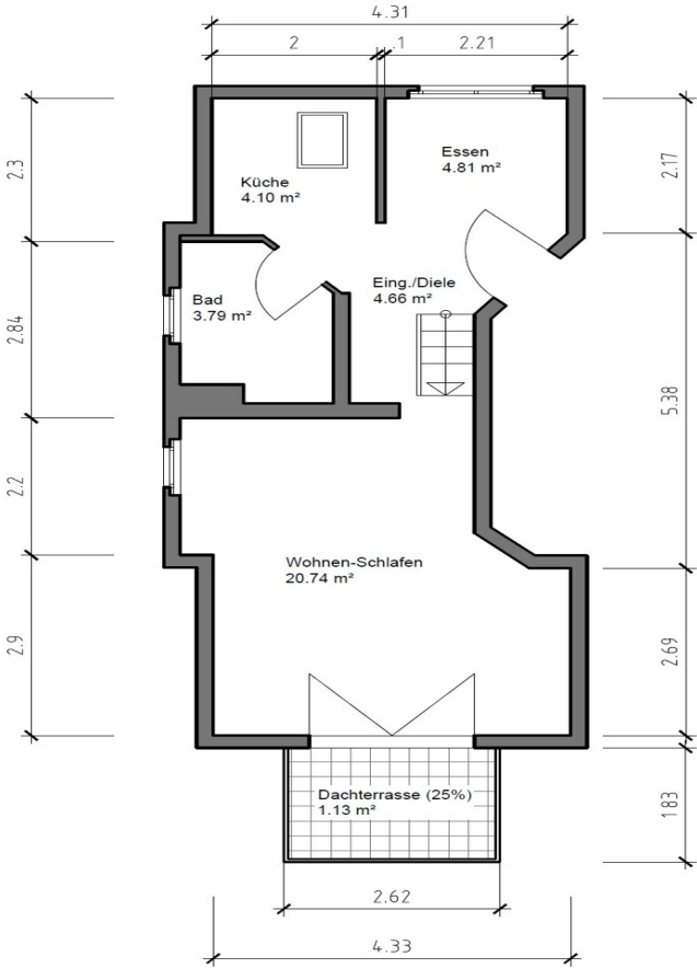
Dachgeschoss
