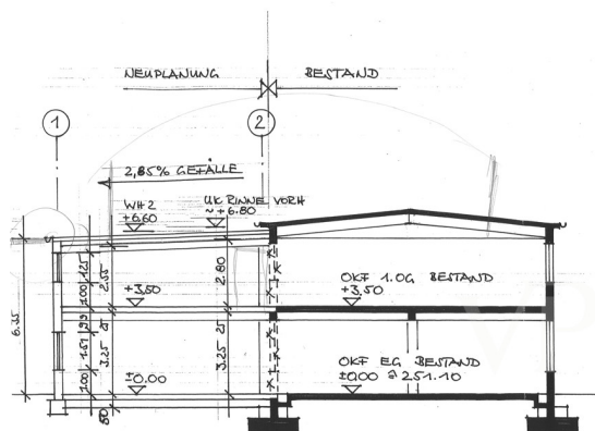
SNITT A-A
