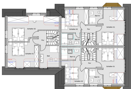
DACHGESCHOSS M 1:100
