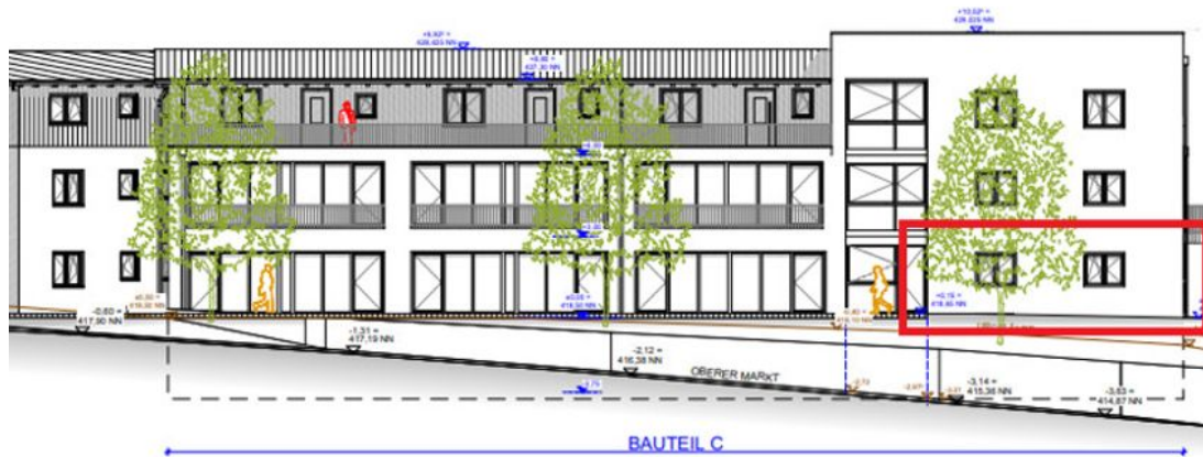
ANSICHT NORD
