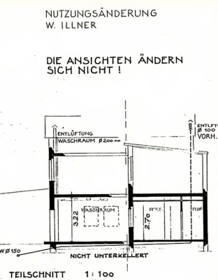
TEILSCHNITT 1:100
