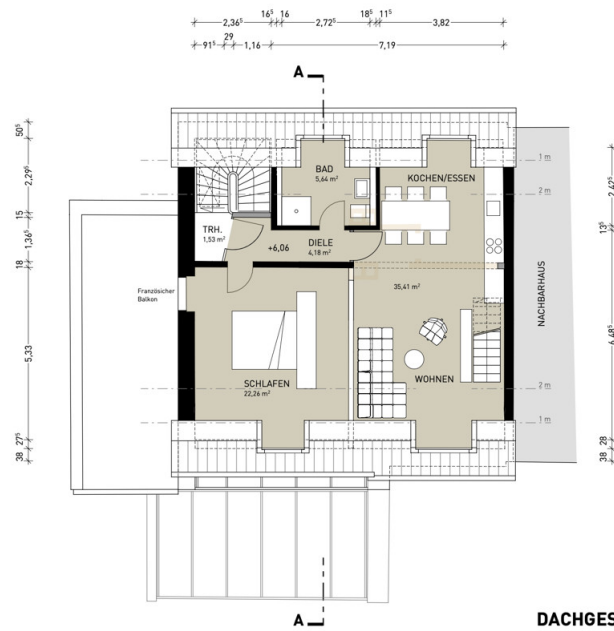
DACHGESCHOSS
