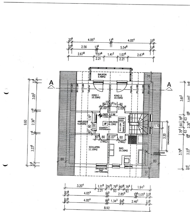
GRUNDRISS OBERGESCHOSS
