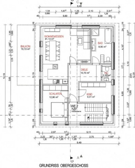
GRUNDRISS OBERGESCHOSS
