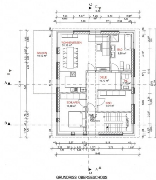
GRUNDRISS OBERGESCHOSS
