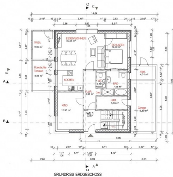
GRUNDRISS ERDGESCHOSS
