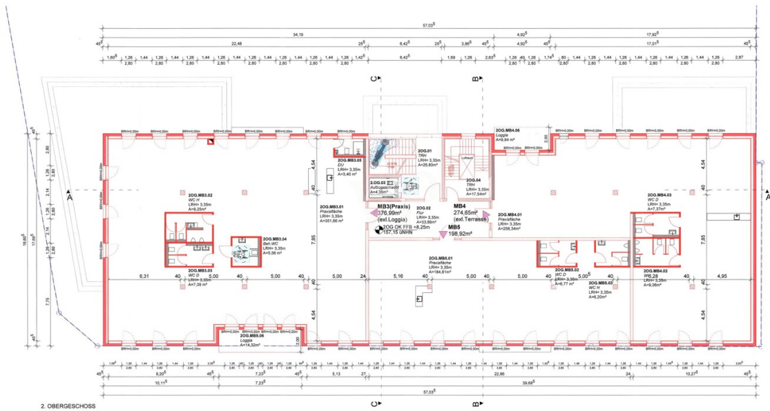
2. OBERGESCHOSS
