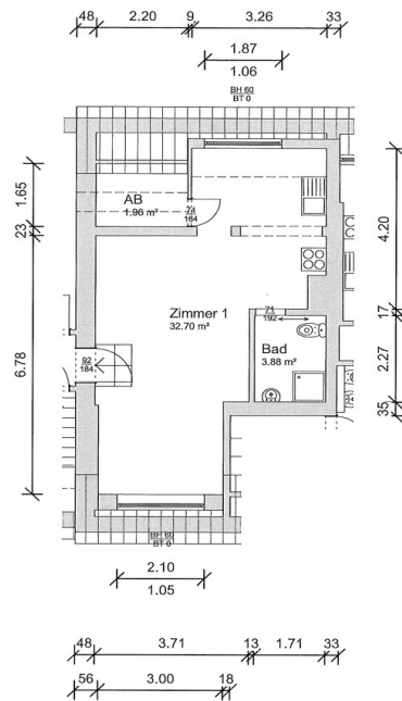
Dachgeschoss: Wohnung 1
