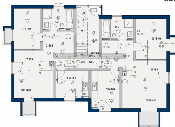
Grundriss EG
