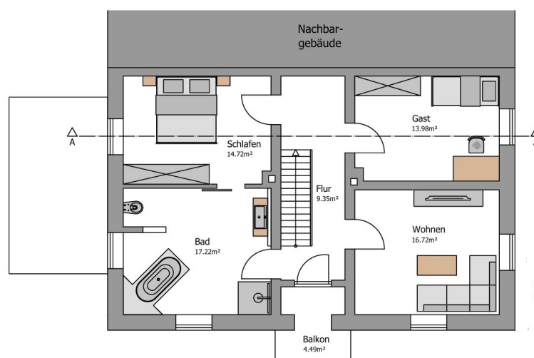
Obergeschoss
