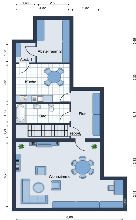
Einliegerwohnung Obergeschoss
