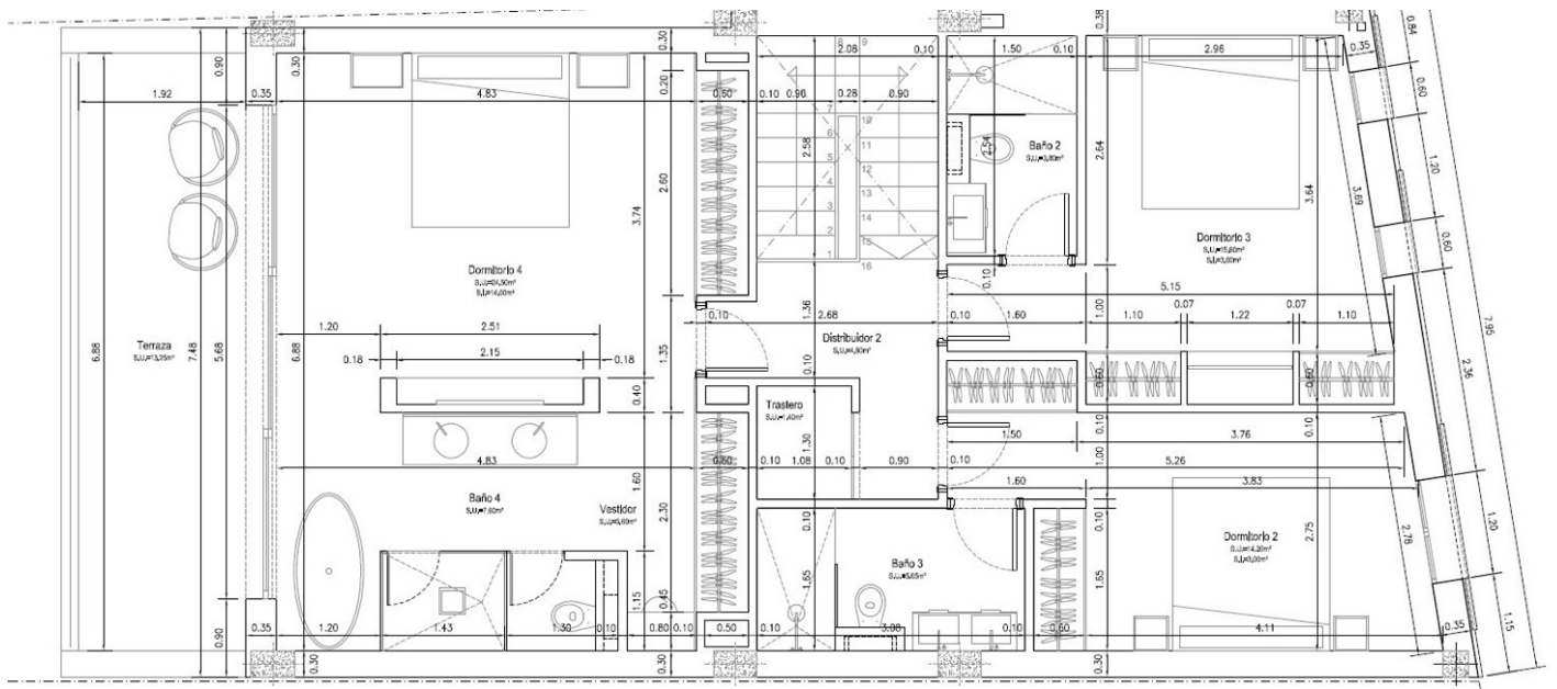
PLANTA PISO
