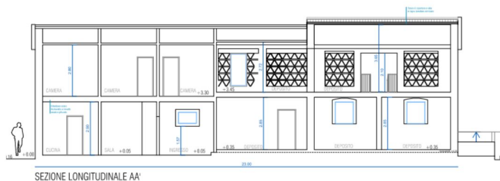
SEZIONE LONGITUDINALE AA'
