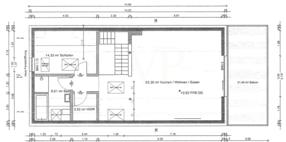
Grundriss OG M 1:100 Entwurf IV
