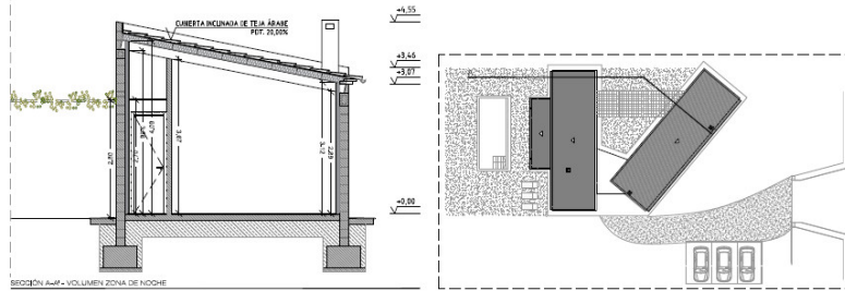
SECCIÓN A-A' - VOLUMEN ZONA DE NOCHE
