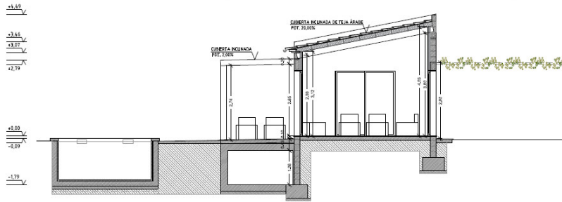
SECCIÓN A-A' - VOLUMEN ZONA DE DÍA
