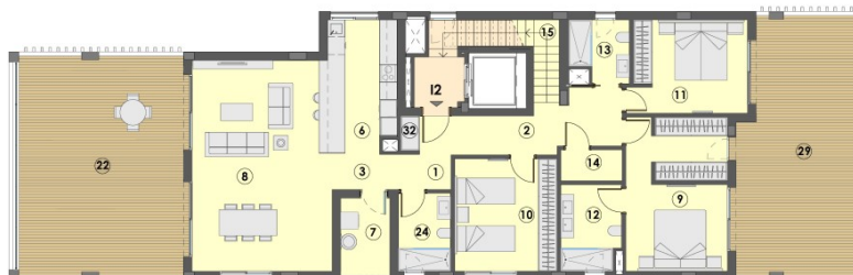
PLANTA SEGUNDA
