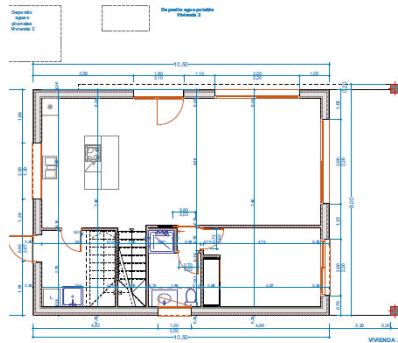
VIVIENDA 2 Planta Sótano
