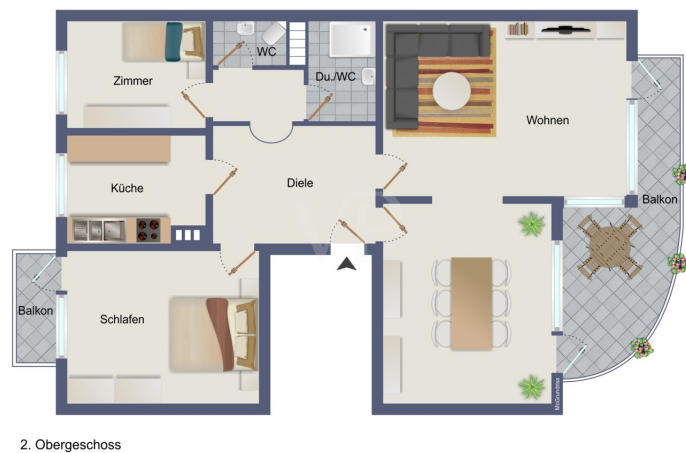
2. Obergeschoss
