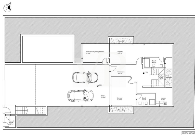
PLANTA SOTANO
