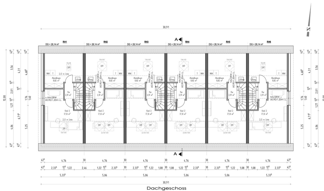
Dachgeschoss
