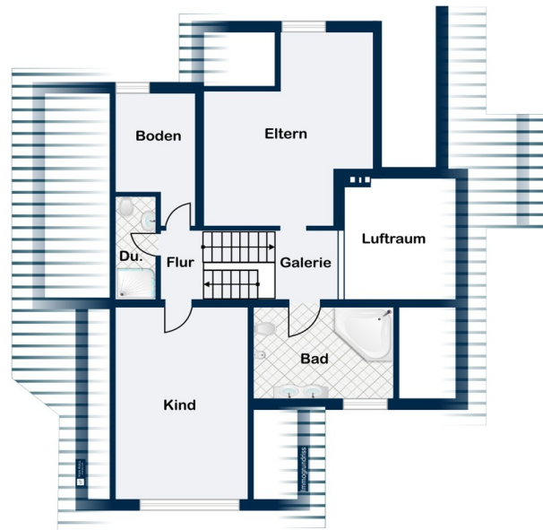
Dachgeschoss
