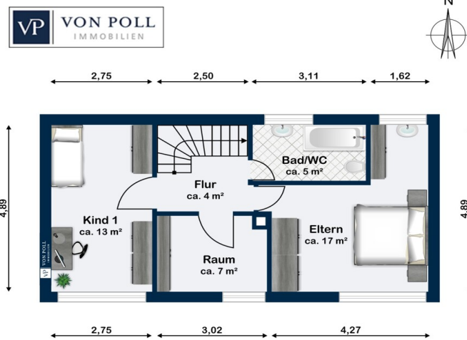
Obergeschoss
