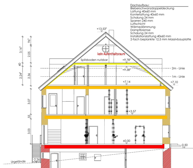
Schnitt A-A
