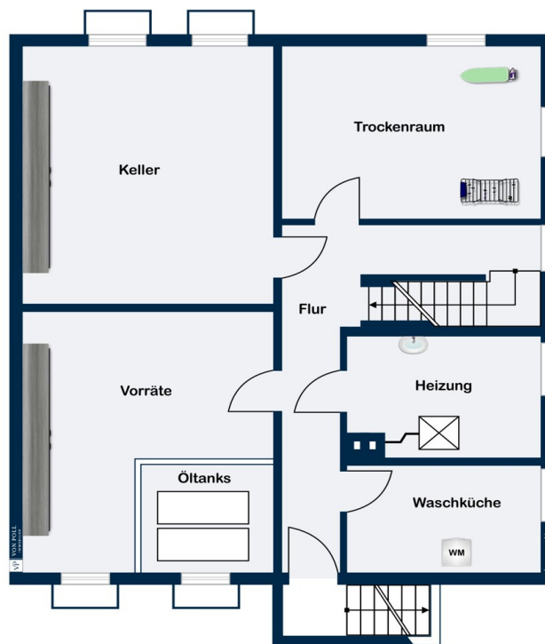
Kellergeschoss
