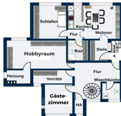
Untergeschoss
