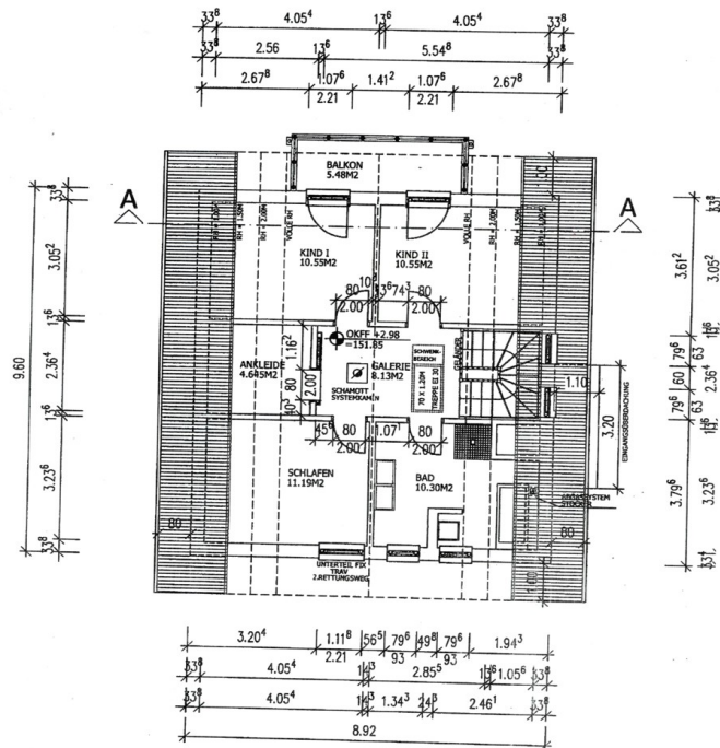
GRUNDRISS OBERGESCHOSS
