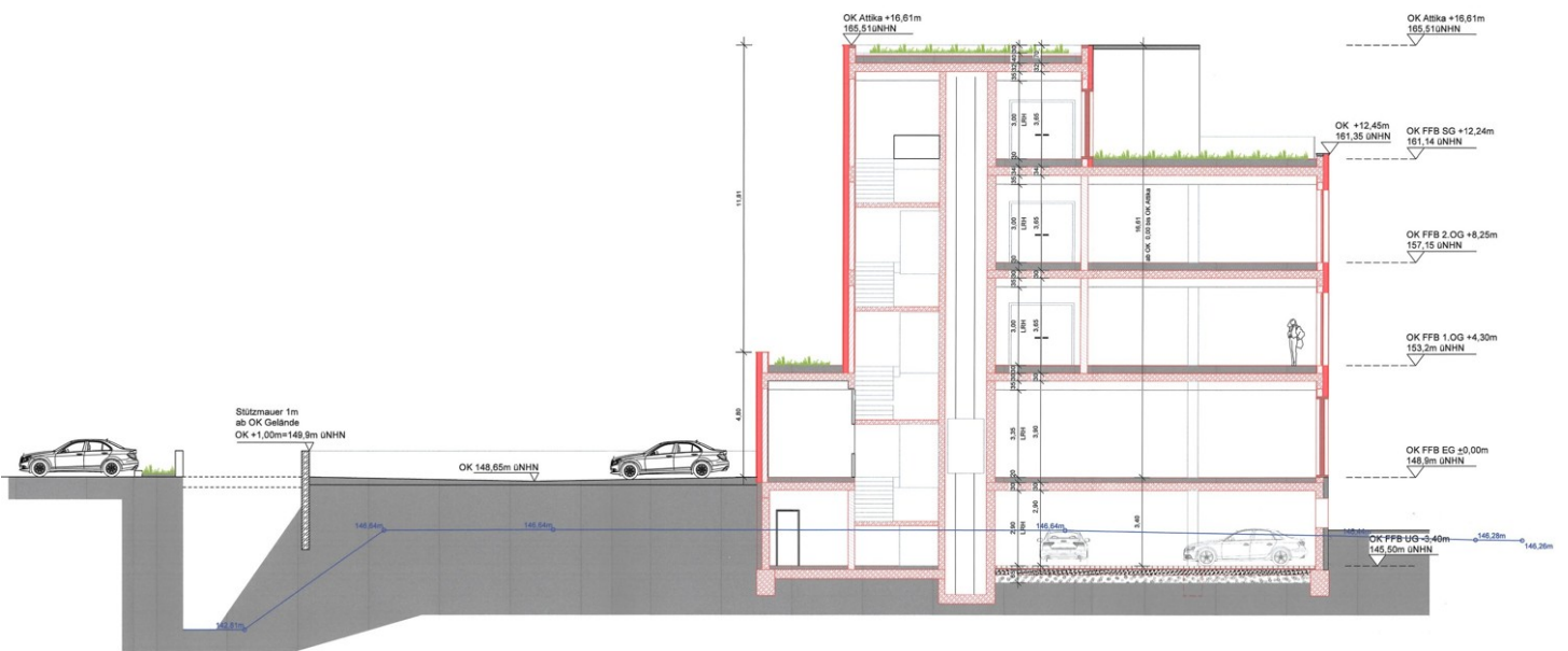
Schnitt C-C
