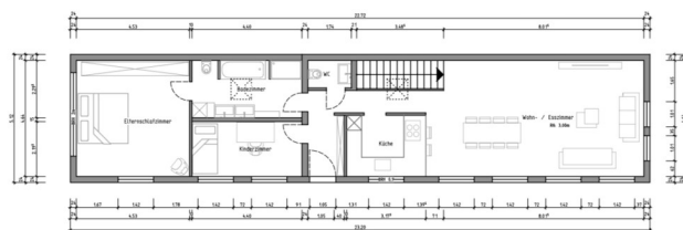
OBERGESCHOSS
