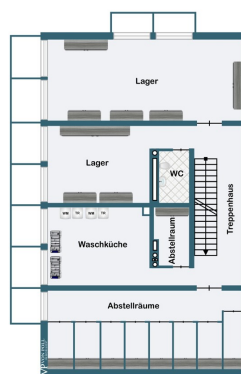
Untergeschoss
