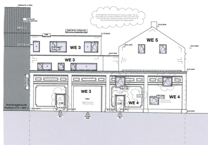
Ansicht Ost
