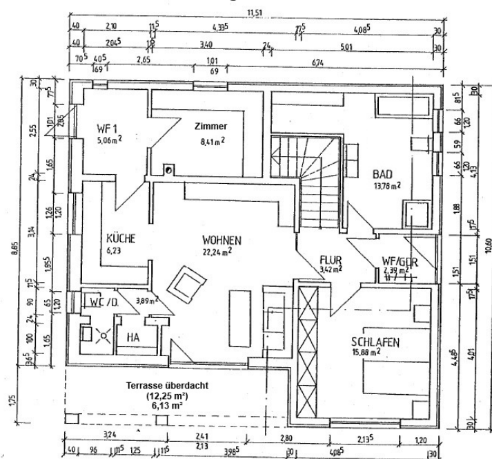
Erdgeschoss
