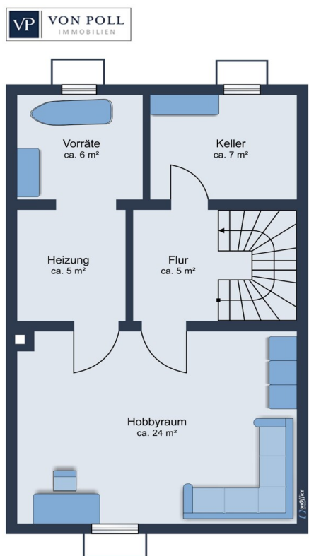
Kellergeschoss
