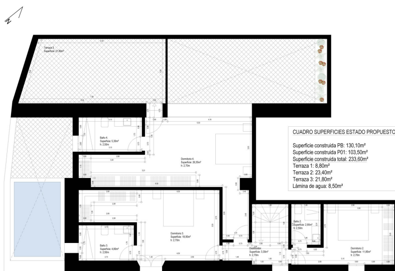
Planta 01. Estado propuesto.
