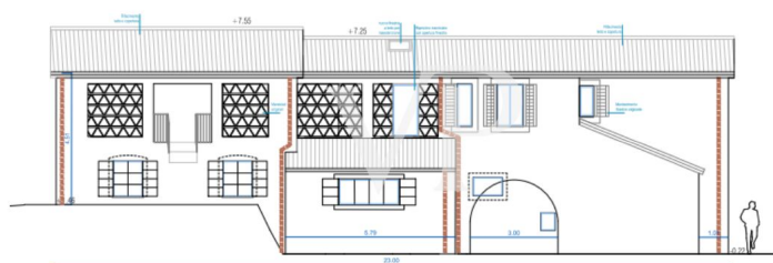
PROSPETTO RETRO
