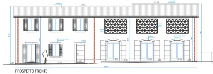
PROSPETTO FRONTE
