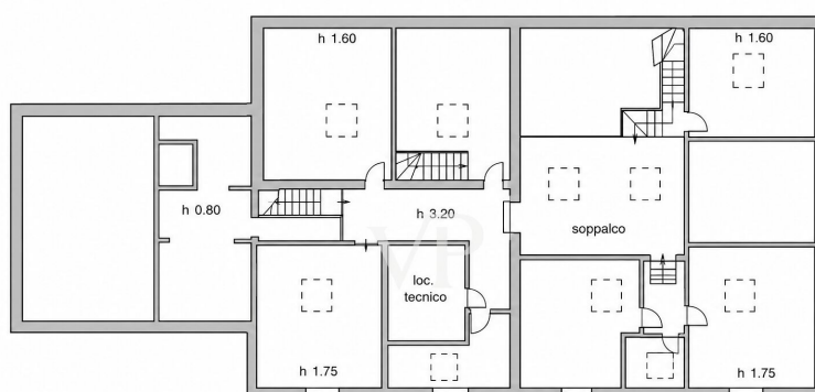
PIANO SOTTOTETTO
