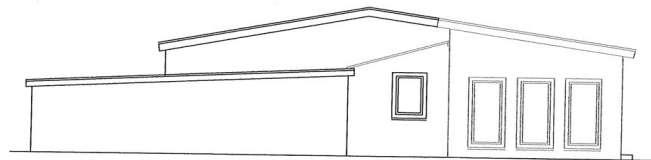
Ansicht - West
