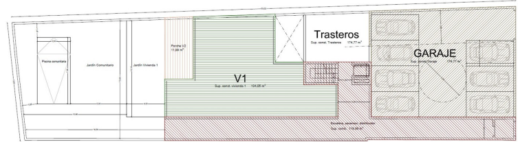
PLANTA BAJA Sup. total: P.B. 445,27 m² Sup. jardín: P.B. 16,54 m² Total: Sup. P.A. 461,81 m²
