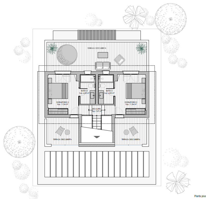
Planta piso
