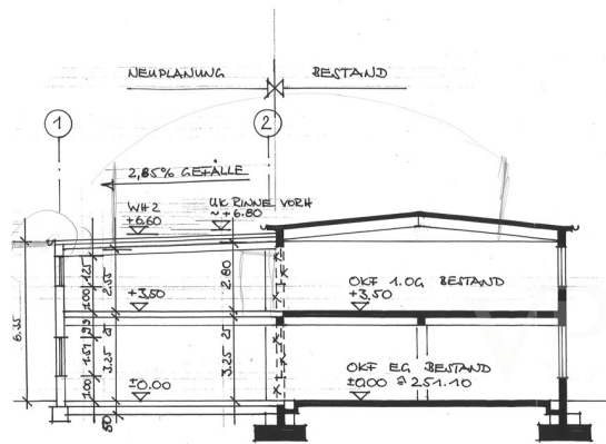
SCHNITT A-A
