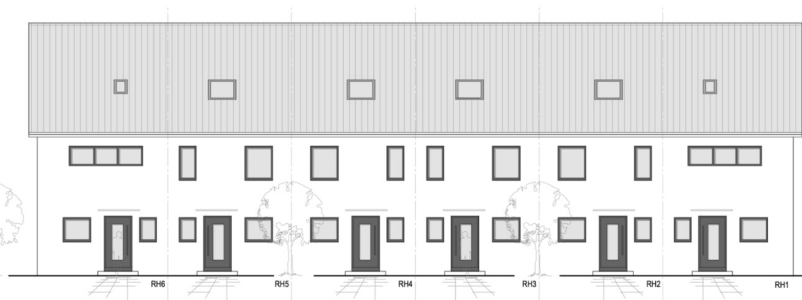
Nord - Ansicht
