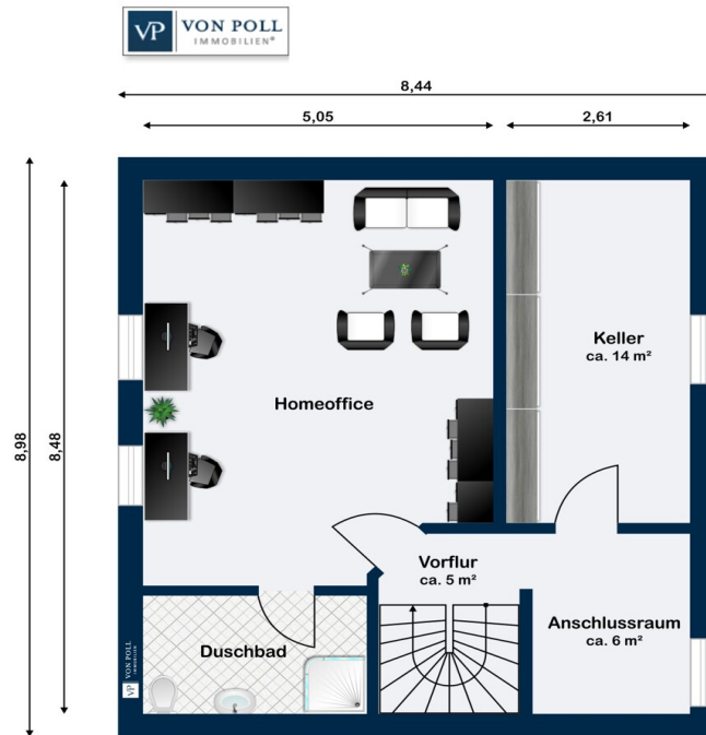
Kellergeschoss
