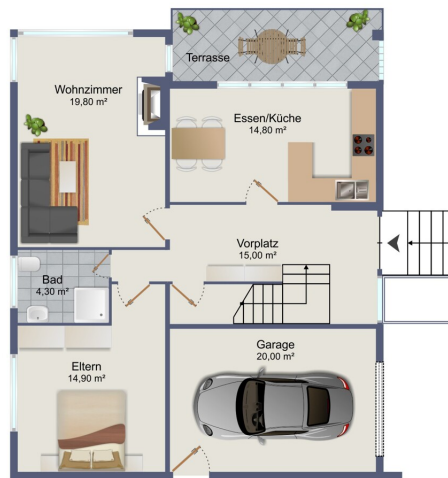
Erdgeschoss
