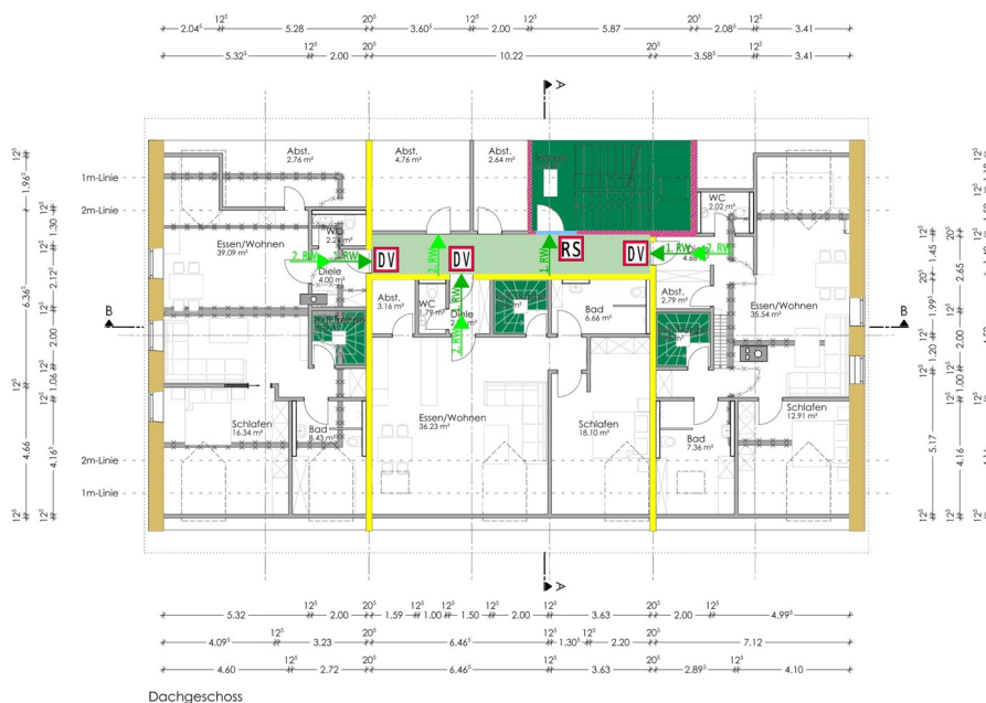
Dachgeschoss
