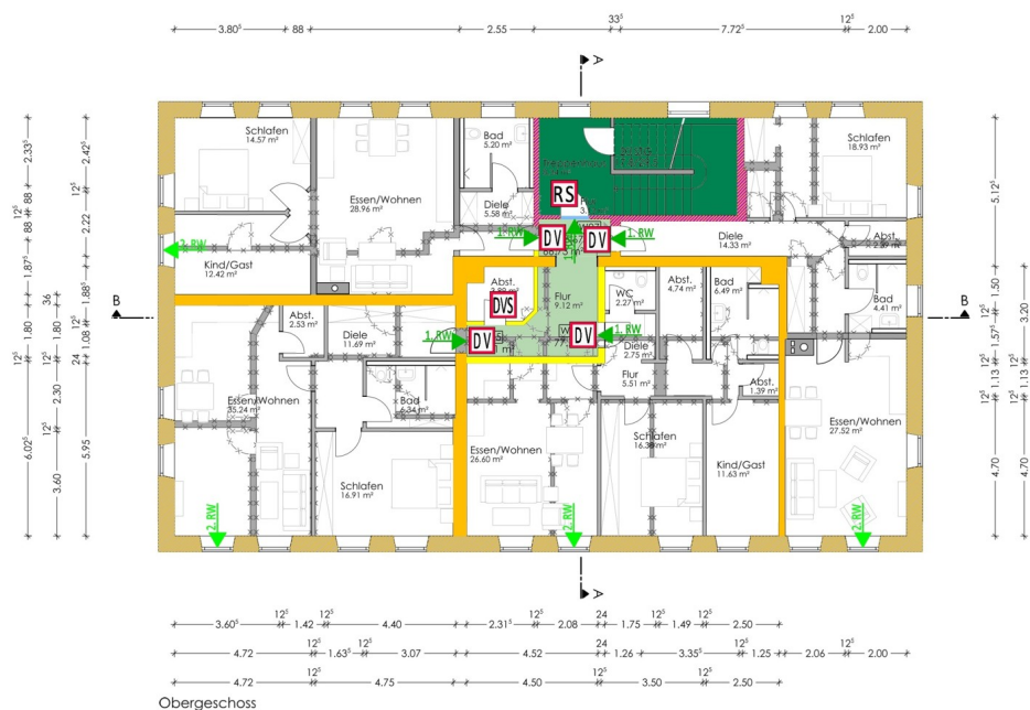
Obergeschoss
