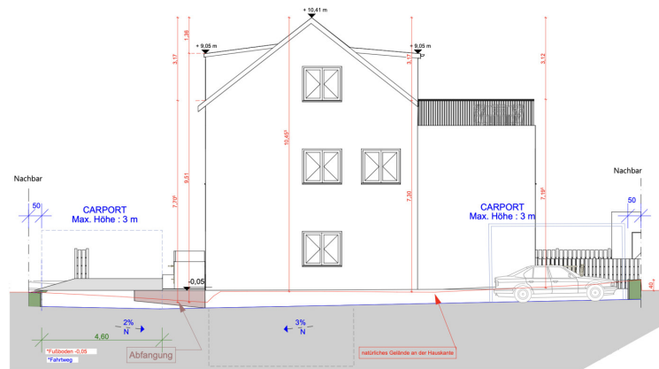
Ansicht NORD-vorderes Haus M 1.100
