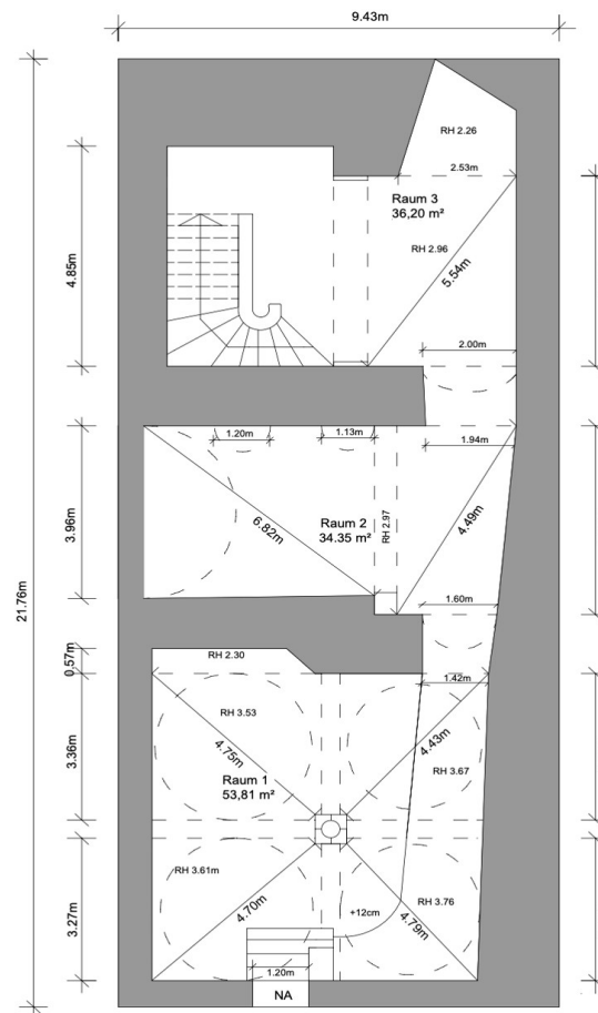
Grundriss KG 1:100
