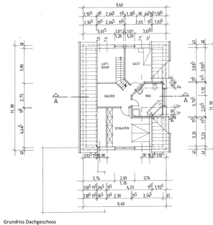
Grundriss Dachgeschoss
