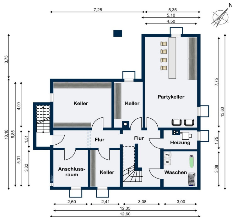
Kellergeschoss
